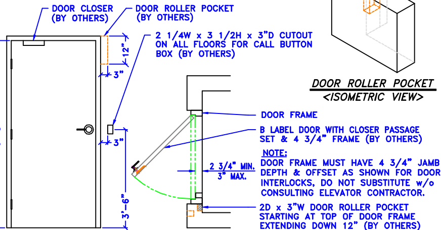
DOOR ELEVATION DOOR FRAME DETAIL
